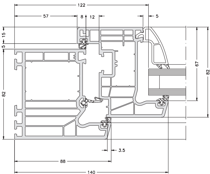
Blendrahmen 82/88 8809 . .
