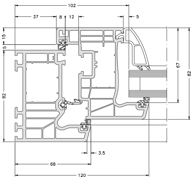
Blendrahmen 82/68 8808 . .
