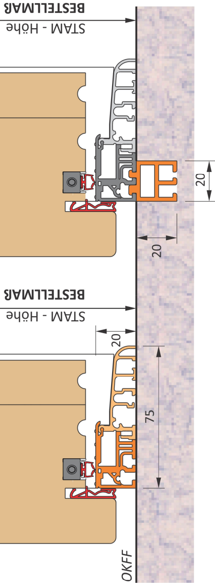
Thermisch getrenntes Profil TB75
