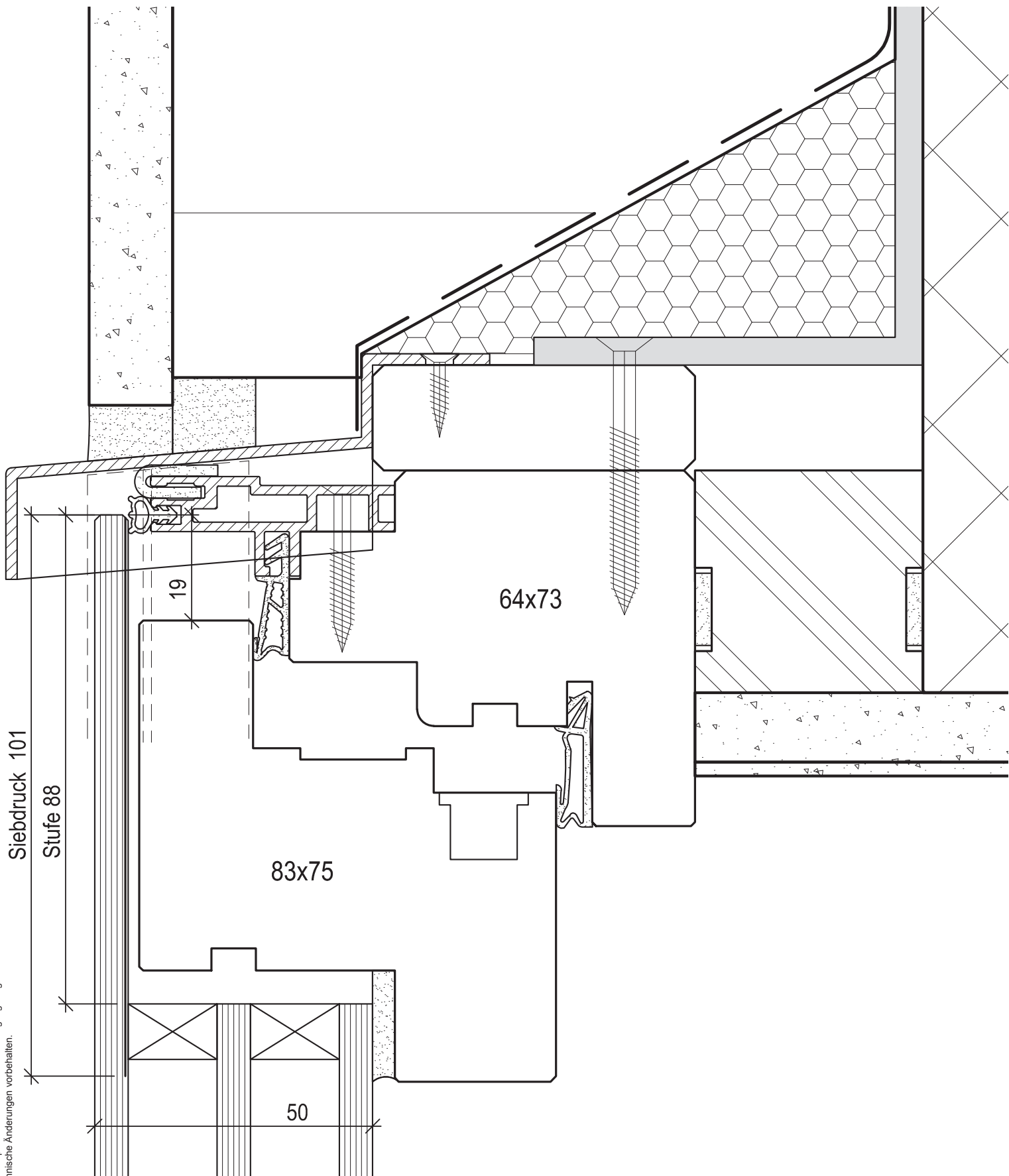
Rahmen oben
