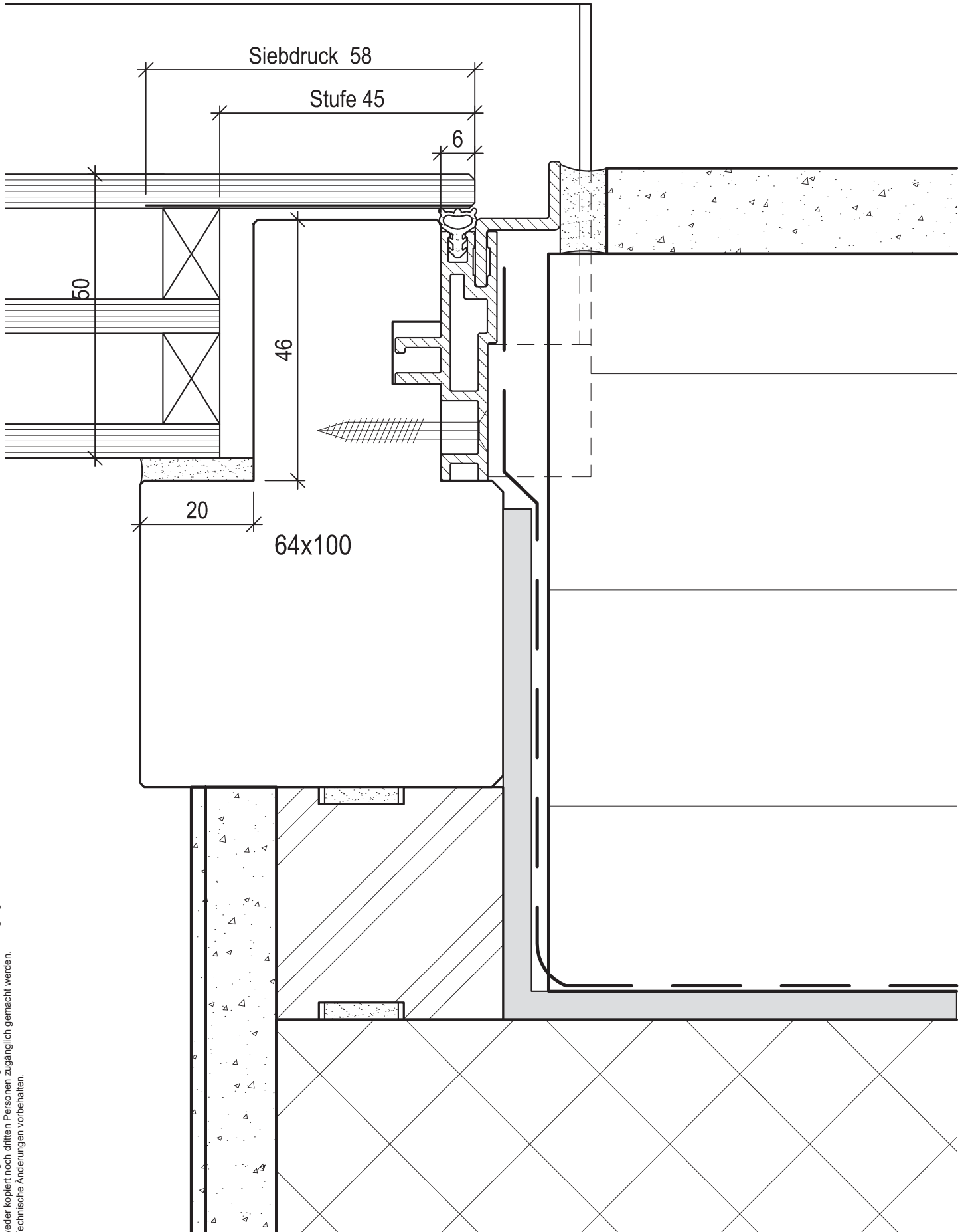
Rahmenverglasung seitlich
